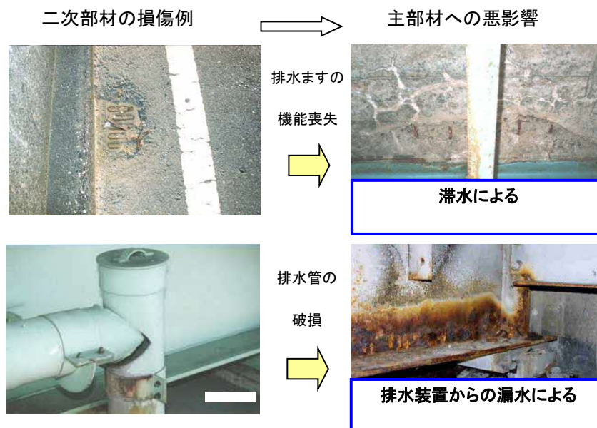
図ー1 二次部材の損傷が主部材へ悪影響を及ぼす例
